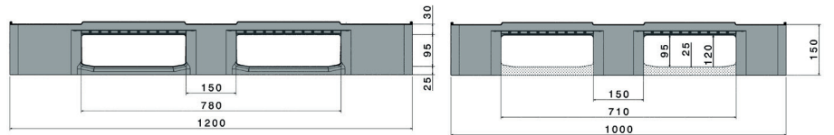
Zeichnung zeigt 7 mm Kantenversion
